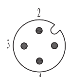
-C3 -D3: 4 pin M12
