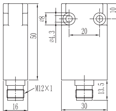
-C3 -D3: 4 pin M12
