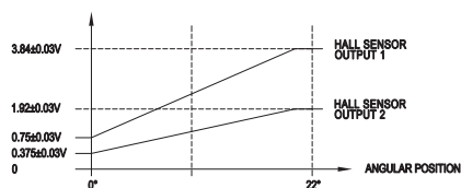
输出特性
